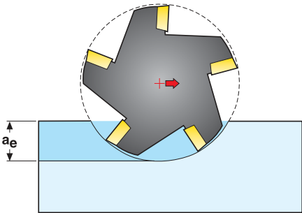
Боковое фрезерование
