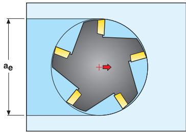
Фрезерование пазов
