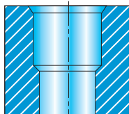
Е1. Расточной инструмент одного диаметра
