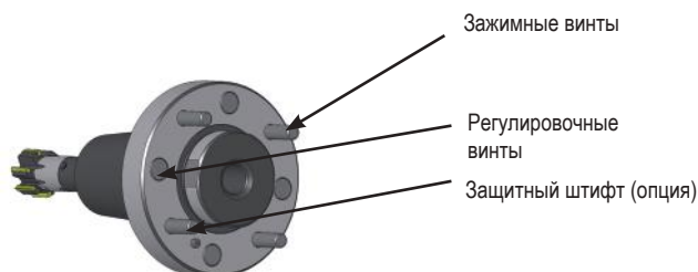
Зажимные винты
